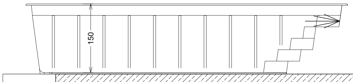
Fundamentplatte armiert laut örtlichen Bodenverhältnissen Foundation slab, reinforced according to the local ground condition
