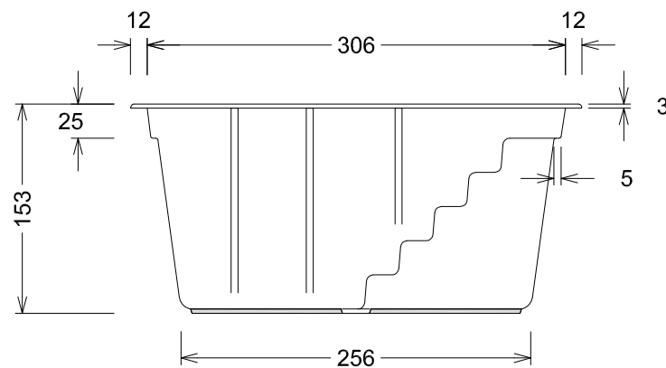
Ansicht Treppenseite - View stair side
