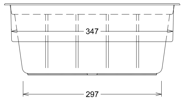
Ansicht Skimmerseite - View skimmer side
