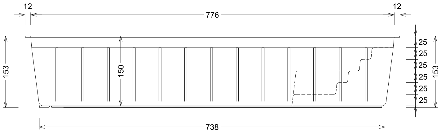
Seitenansicht - Side view
