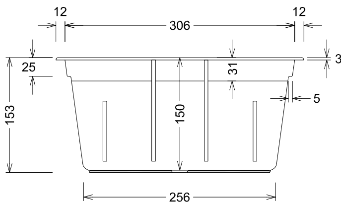
Ansicht Skimmerseite - View skimmer side
