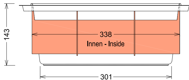
Ansicht Rolloseite - View cover side
